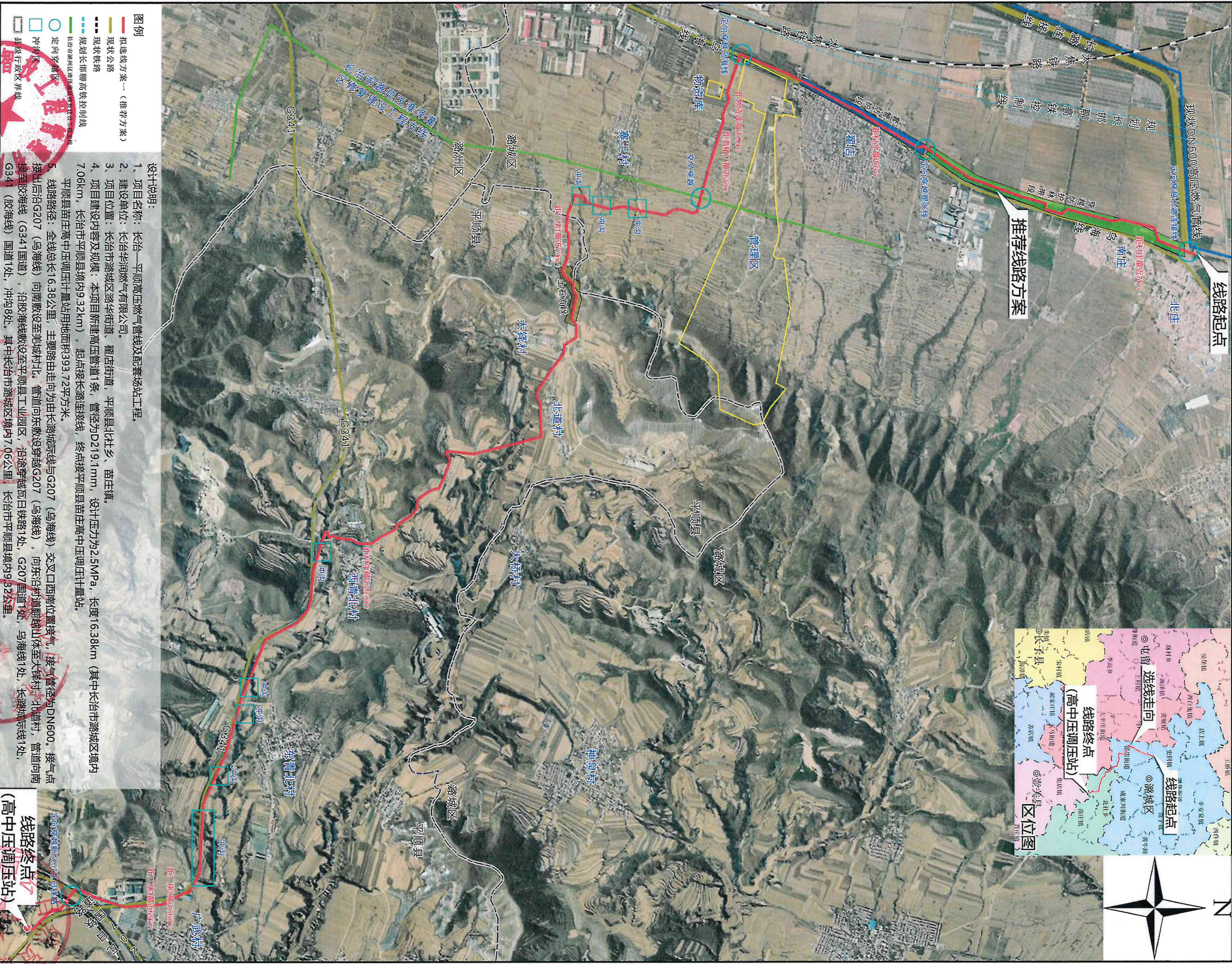
项目推荐选线及高中压调压站选址方案图
